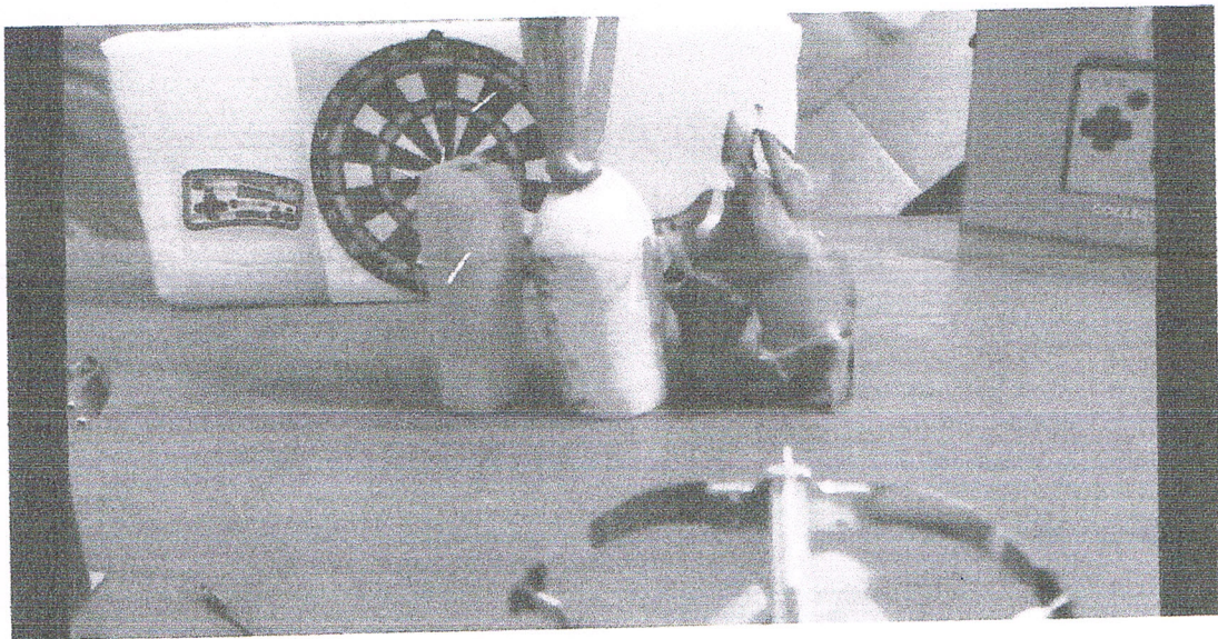
ภาพที่ ๓ ทดสอบการยิงหน้าไม้จิวด้วยไม้จิ้มฟัน ไปยังผัก ผลไม้ รวม ๓ ชนิด ได้แก่ แครอท หัวไชเท้า และแก้วมังกร
